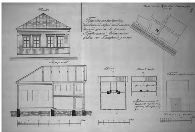
Проект на постройку деревянной еврейской молитвенной школы. НИАБ. Ф. 3209. Оп. 1. Ед.хр. 1683. Л.7
