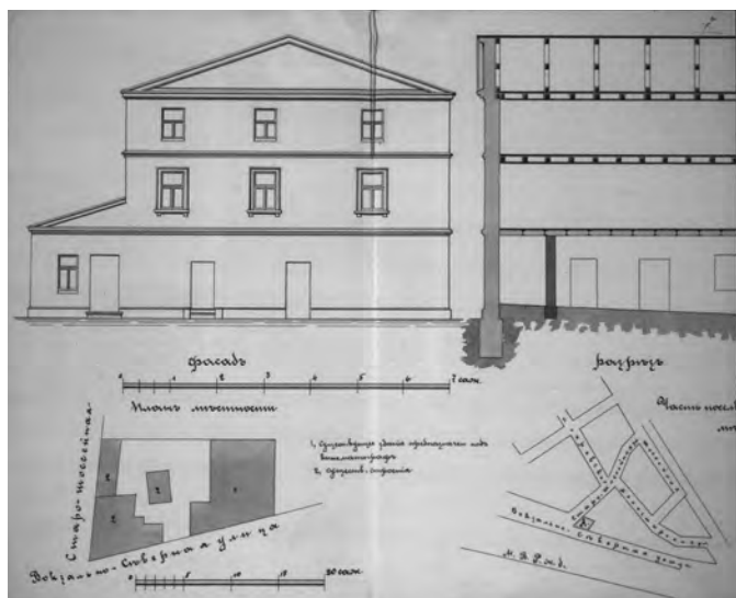
Проект на устройство кинематографа. НИАБ. Ф. 3209. Оп. 1. Д. 1796. Л. 7, 8
