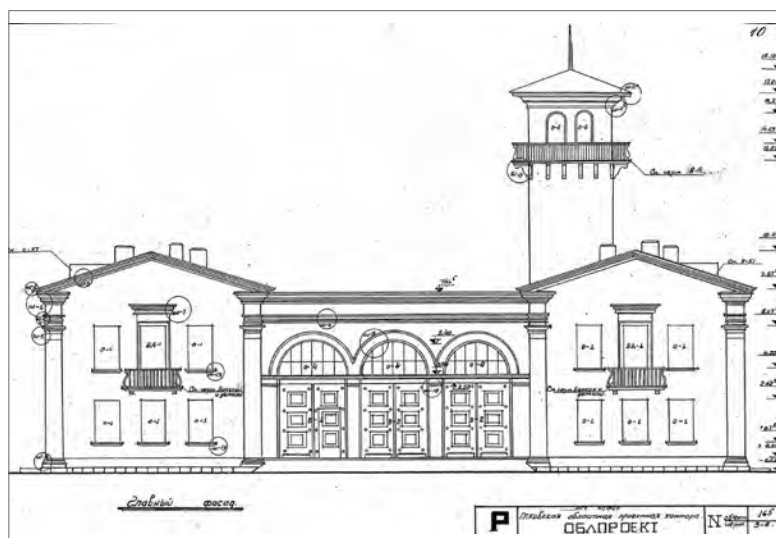
Рис. 10. Рабочий проект здания пожарной части в Порхове. Главный фасад (ГАПО, ф.Р-1924, оп. 1, д. 394, л. 10-а)
