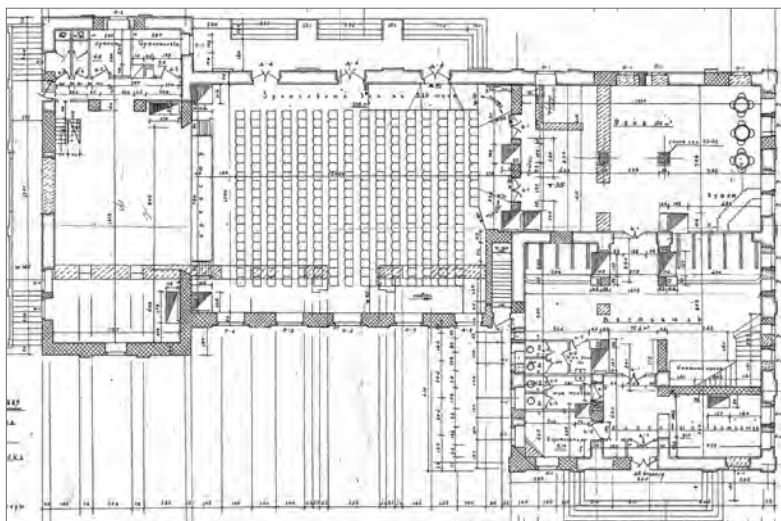
Рис. 5. План первого этажа Порховского дома культуры. Фрагмент. (ГАПО, ф.Р-1924, оп. 1, д. 111, лист 4)
