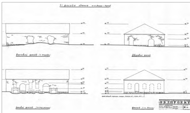
Рис. 12. Обмерные чертежи фасадов здания, реконструируемого под универмаг (ГАПО, там же)
