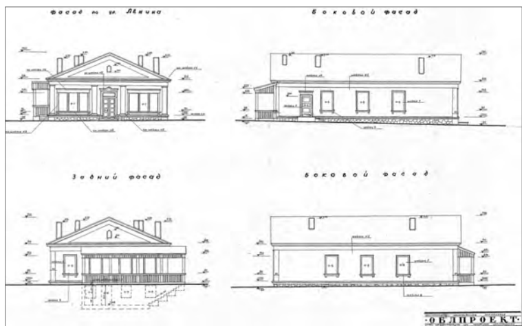
Рис. 15. Рабочий проект (фасады) здания порховского универсама (ГАПО, там же)
