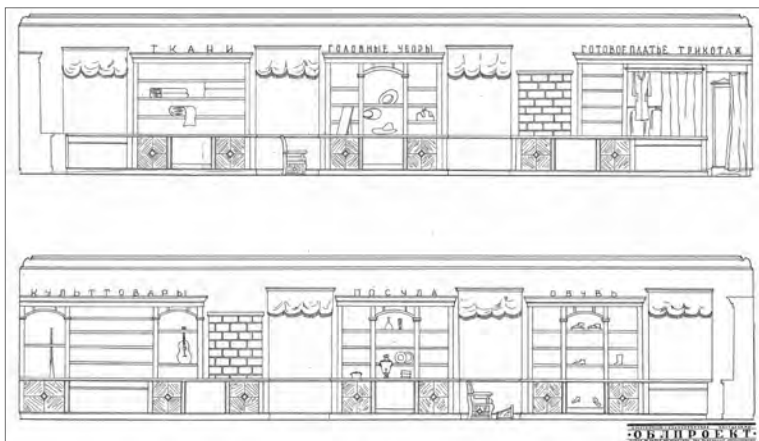
Рис. 16. Проектные развёртки стен торгового зала порховского универсама (ГАПО, там же, л. 11)
